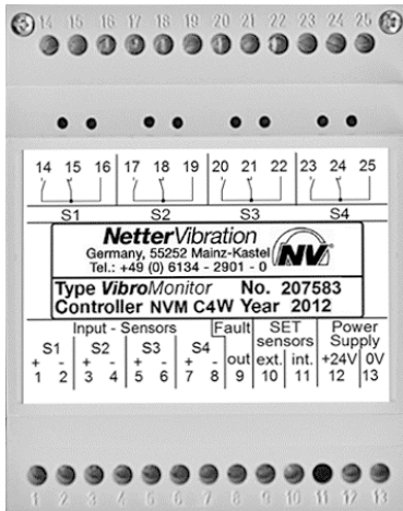
Klemmenbelegung NVM C4W
