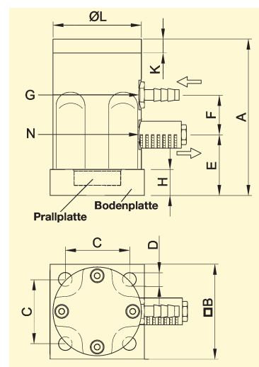
NTP 32 und NTP 48 B+C
