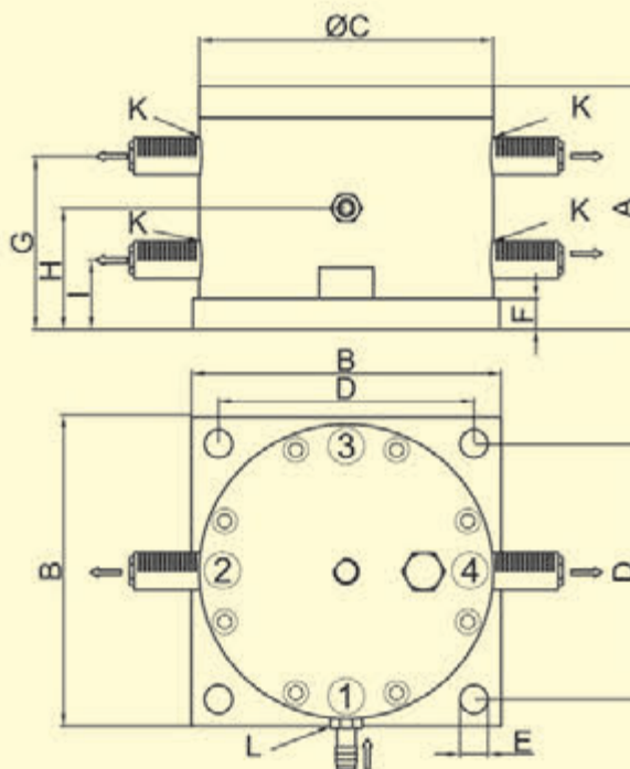
Gehäusety III NTS 21/04 bis NTS 20/40
