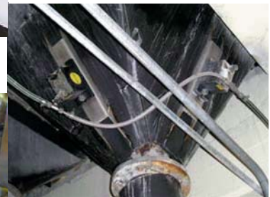
Prévention de la formation de ponts à l'aide de vibrateurs pneumatiques circulaires
