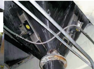
Eliminación de obstrucciones en tolvas y silos mediante vibradores neumáticos rotativos
